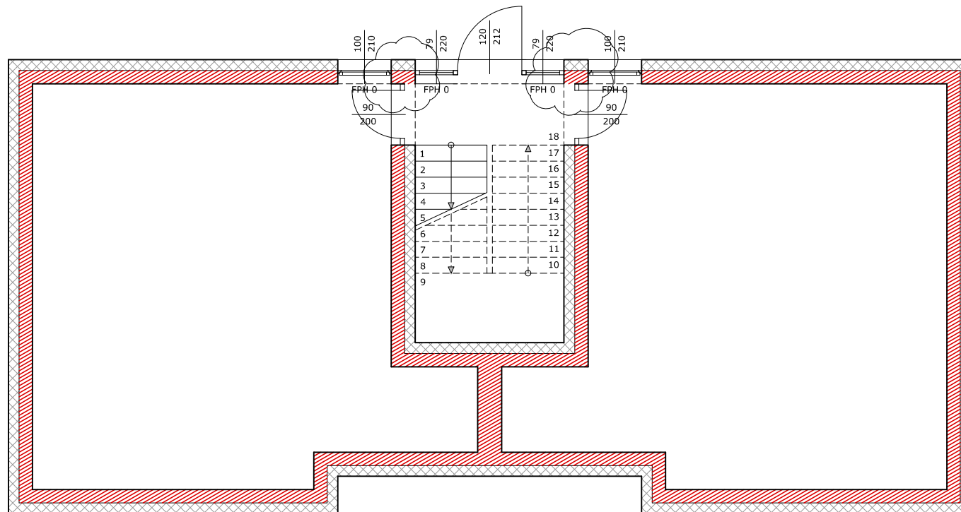
Grundriss M= 1:100
