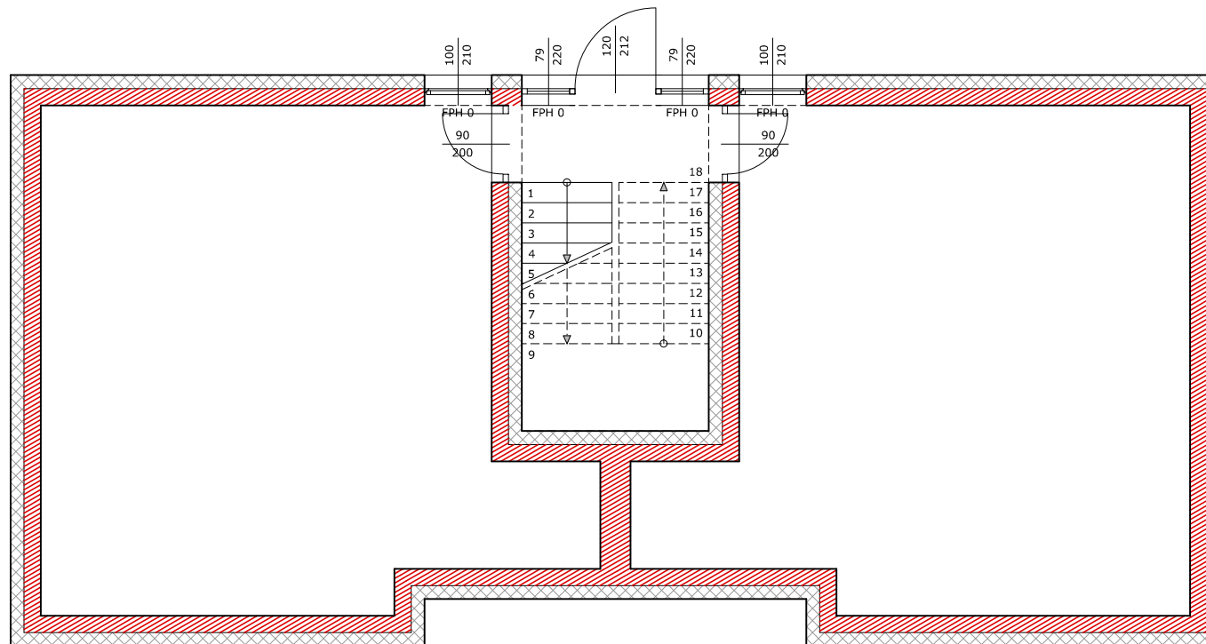
Grundriss M= 1:100
