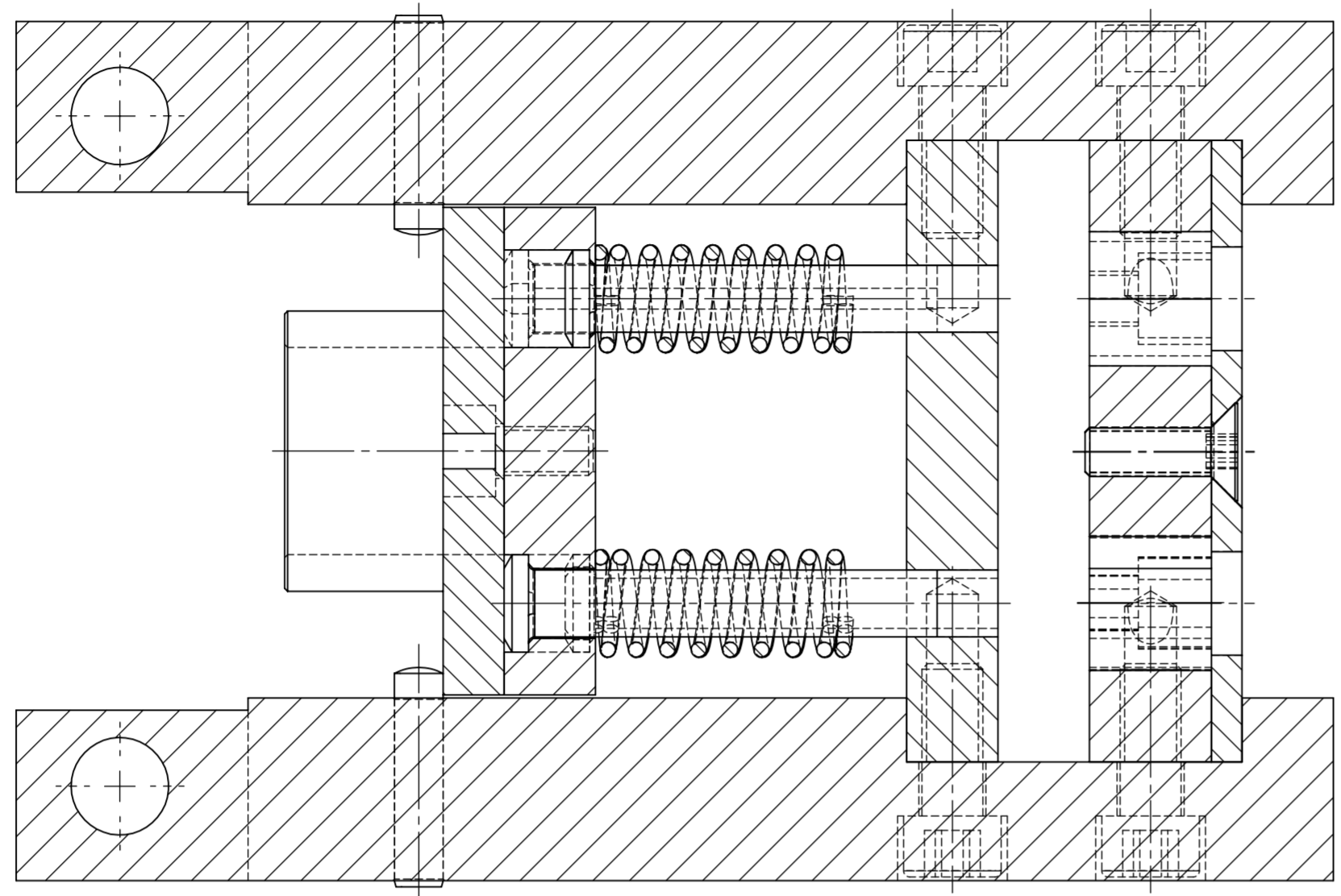
SCHNITT A-A
