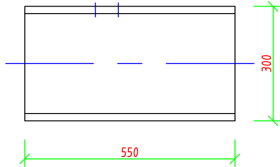
1 HEB 300 1 St. Vorderansicht Maßstab 1:10
