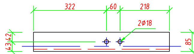
2 U 240 Draufsicht Maßstab 1:10
