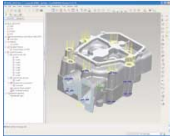
Pro/ENGINEER Advanced Mechanics simuliert durch die Definition von Vorspannbedingungen für Bolzen und internen Verbrennungslasten präzise reale Bedingungen für die Spannungsanalyse.
