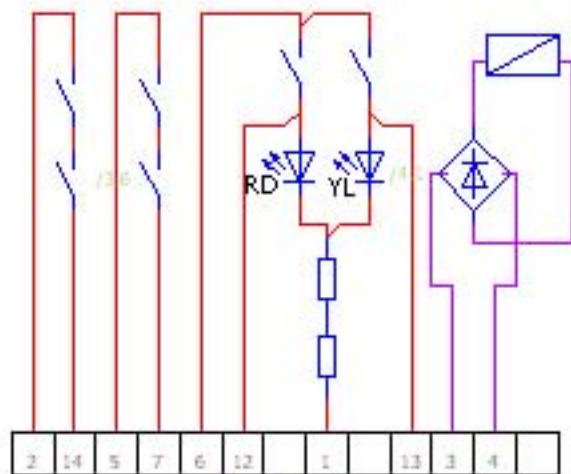
Klemmleiste
