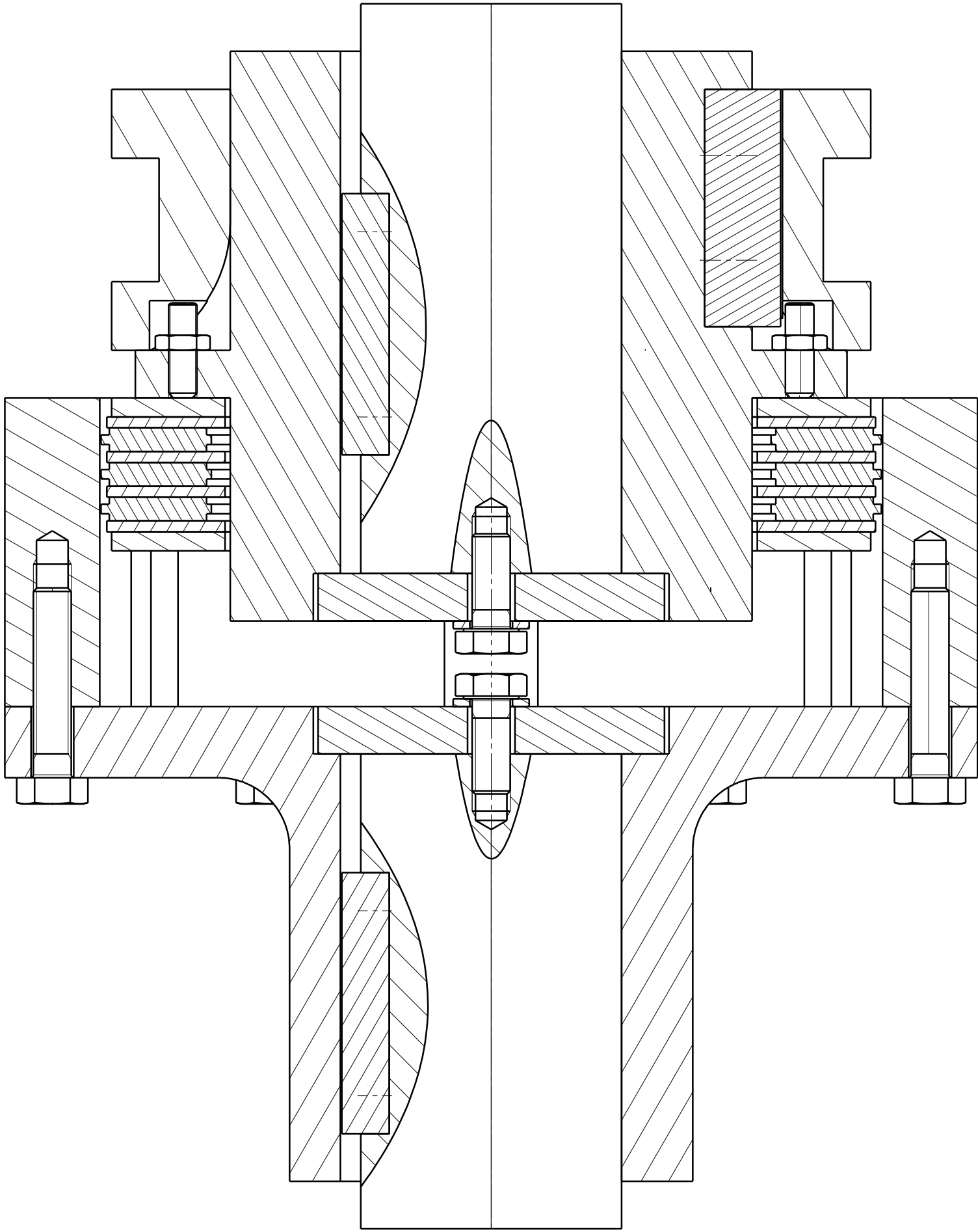
Schnitt A-A Maßstab: 1:1
