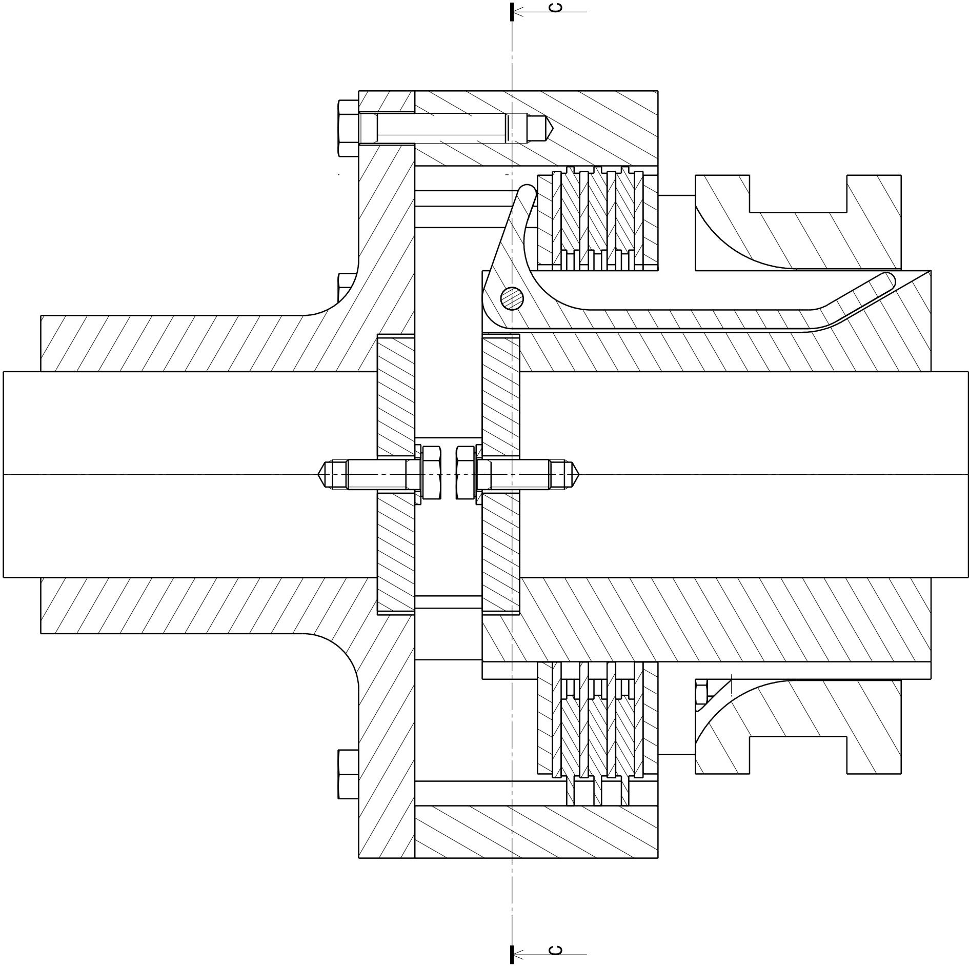
SchnittB-B Maßstab: 1:1
