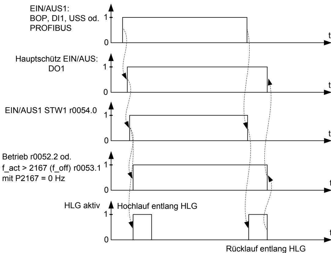
Abbildung 2-2 Zeitlicher Ablauf der Ein- / Ausschaltrihenfolge bei Hauptschützensteuerung für MICROMASTER 430/440
