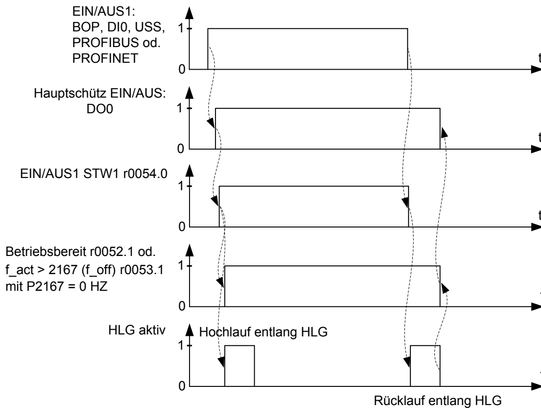
Abbildung 2-3 Zeitlicher Ablauf der Ein- / Ausschaltrihenfolge bei Hauptschützensteuerung für SINAMICS G120 und SINAMICS G120D
