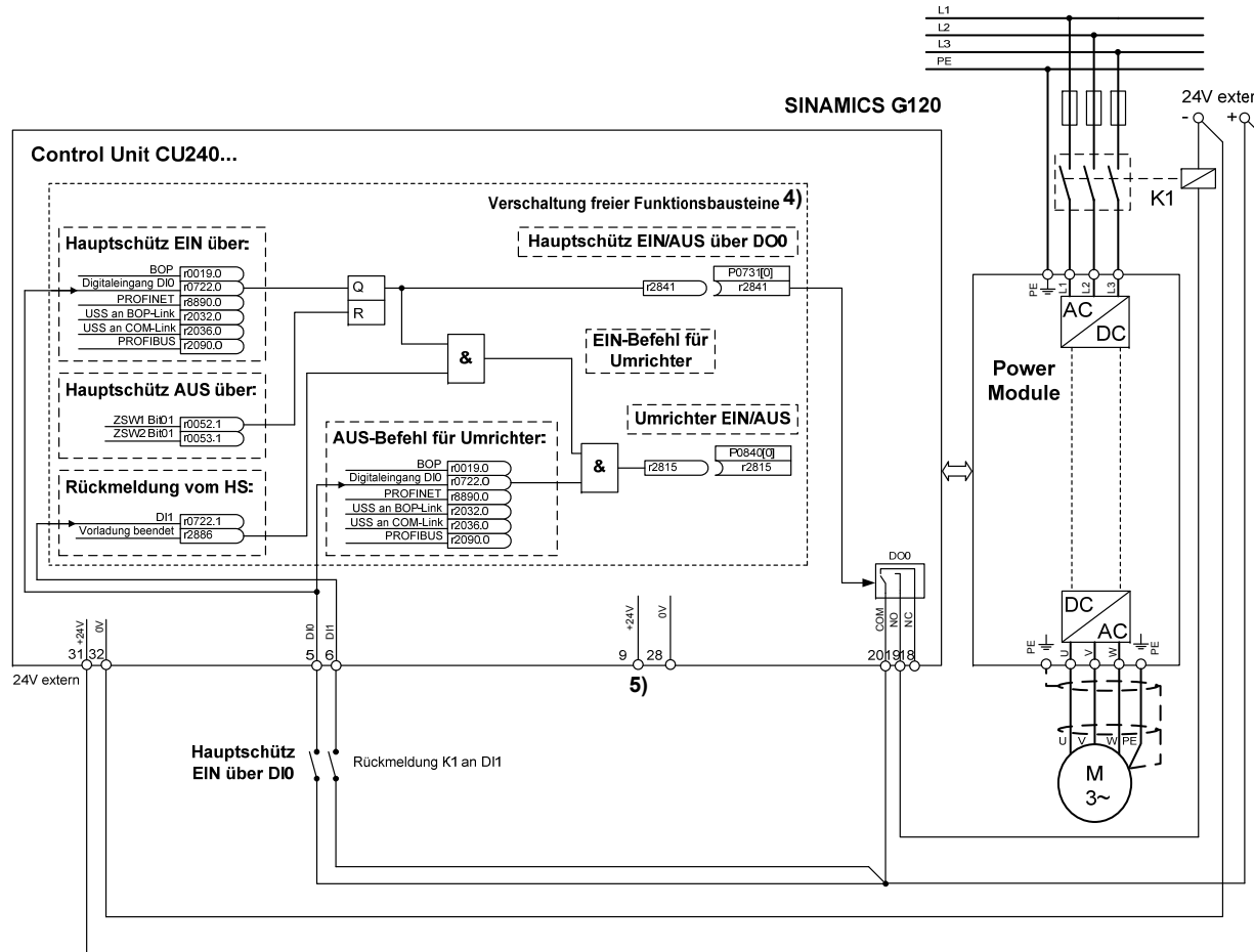
Abbildung 2-5 Hauptschützensteuerung für SINAMICS G120 über DO0: Verschaltung der Klemmen
