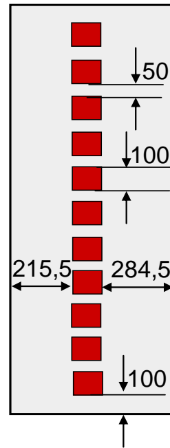
Schnitt A-A
