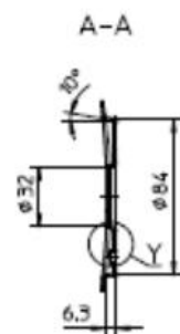
Flanschausführung Model-Nr.: 1479162
