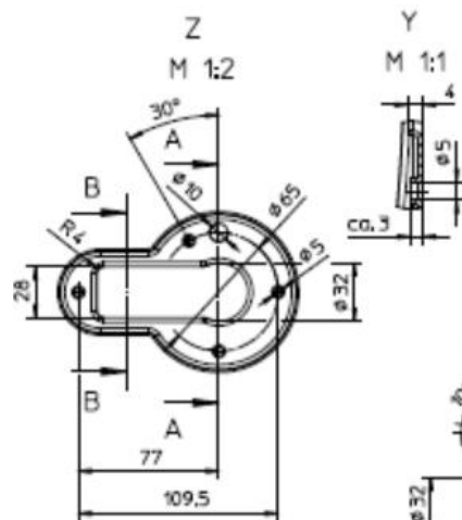
Flanschausführung Model-Nr.: 1479162
