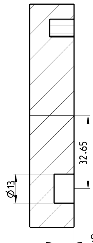
Projektionsansicht voll ausgerichteter Querschnitt B-B
