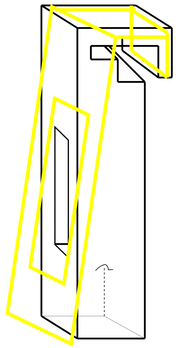
Schalenmodell
