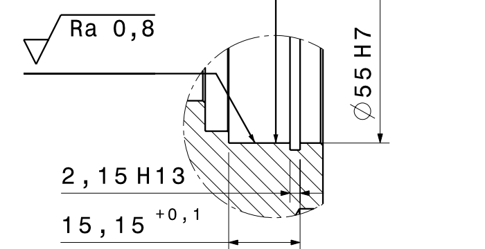
Detail A Maßstab 1:1
