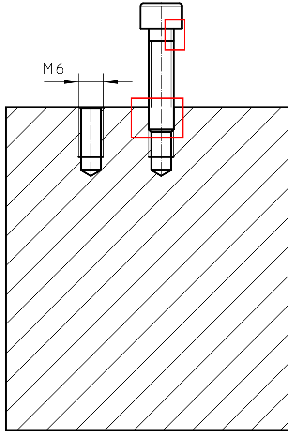
Schnitt B-B
