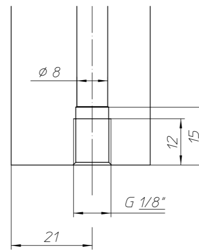
SCHNITT A-A
