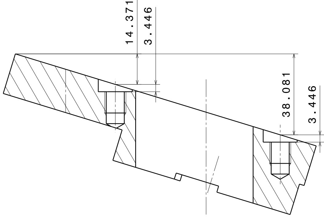
Schnittansicht B-B Maßstab: 1:1
