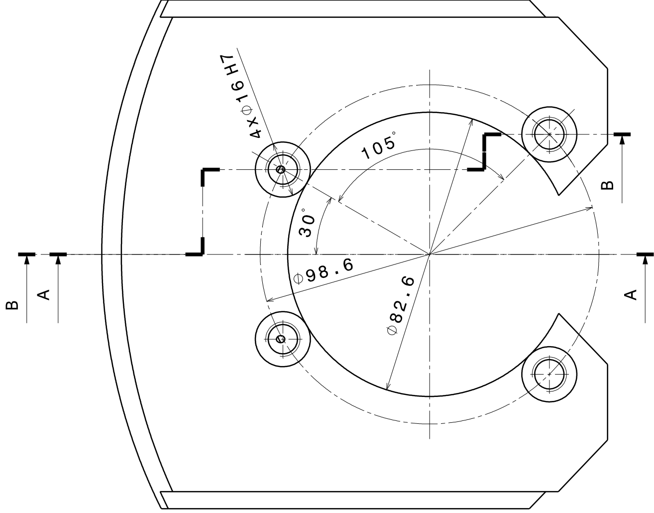
Draufsicht Maßstab: 1:1
