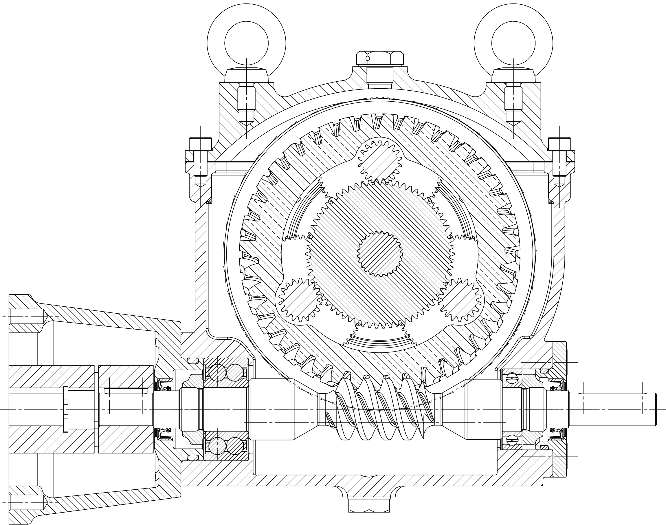
SNITT-DARSTELLUNG B-B MAßSTAB 1 : 1
