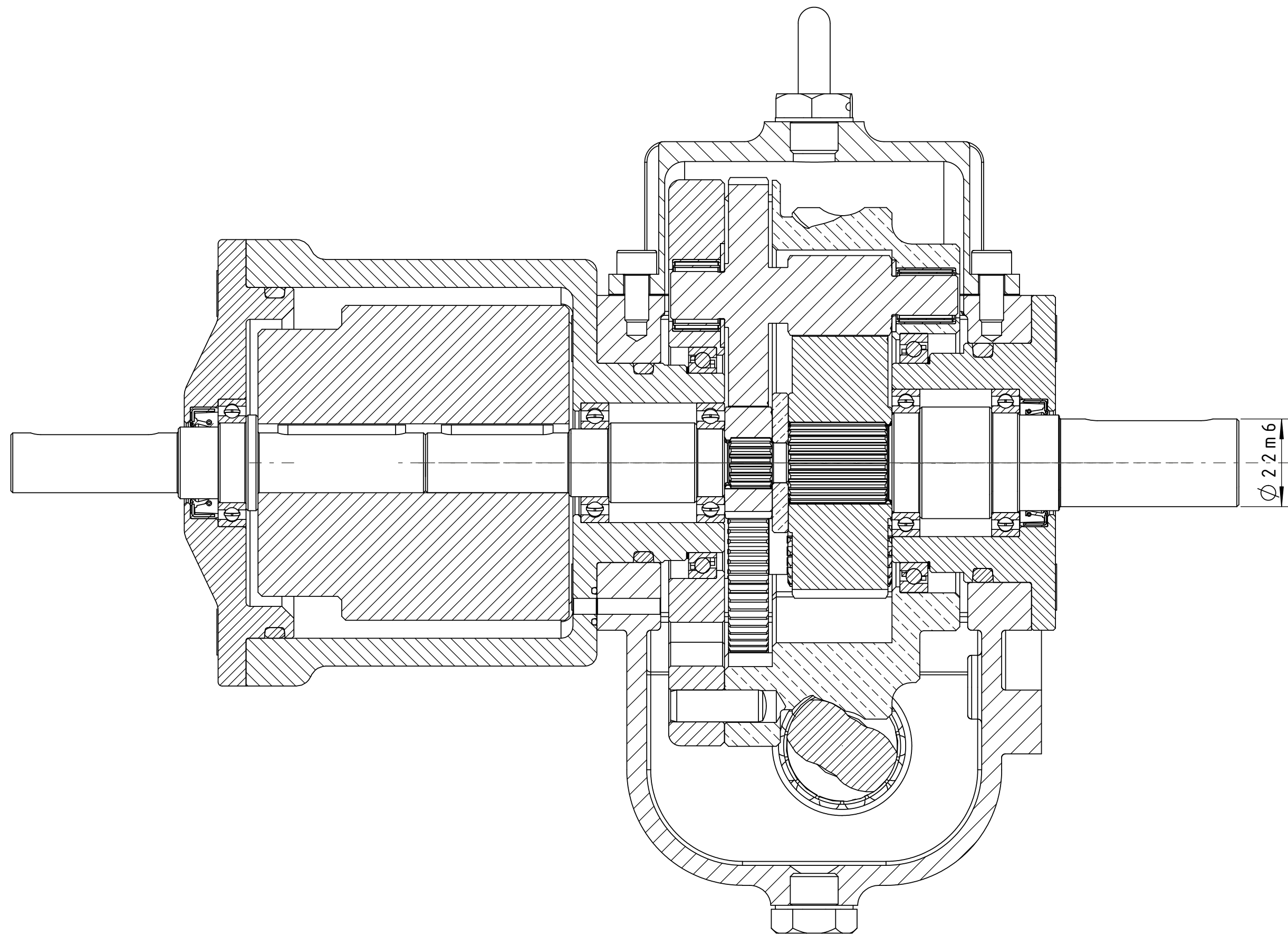
SNITT-DARSTELLUNG A-A MAßSTAB 1 : 1
