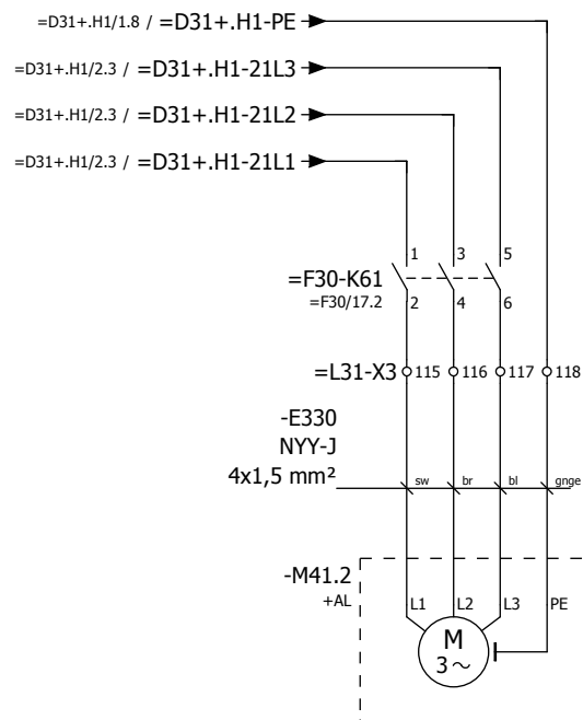
Bremse Antriebsseite - Links
