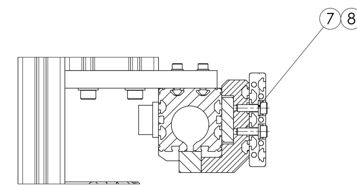
A-A (1 : 2)
