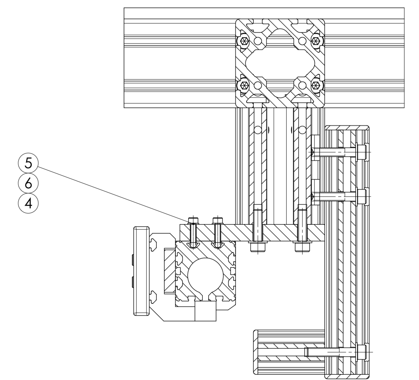
C-C (1 : 2)
