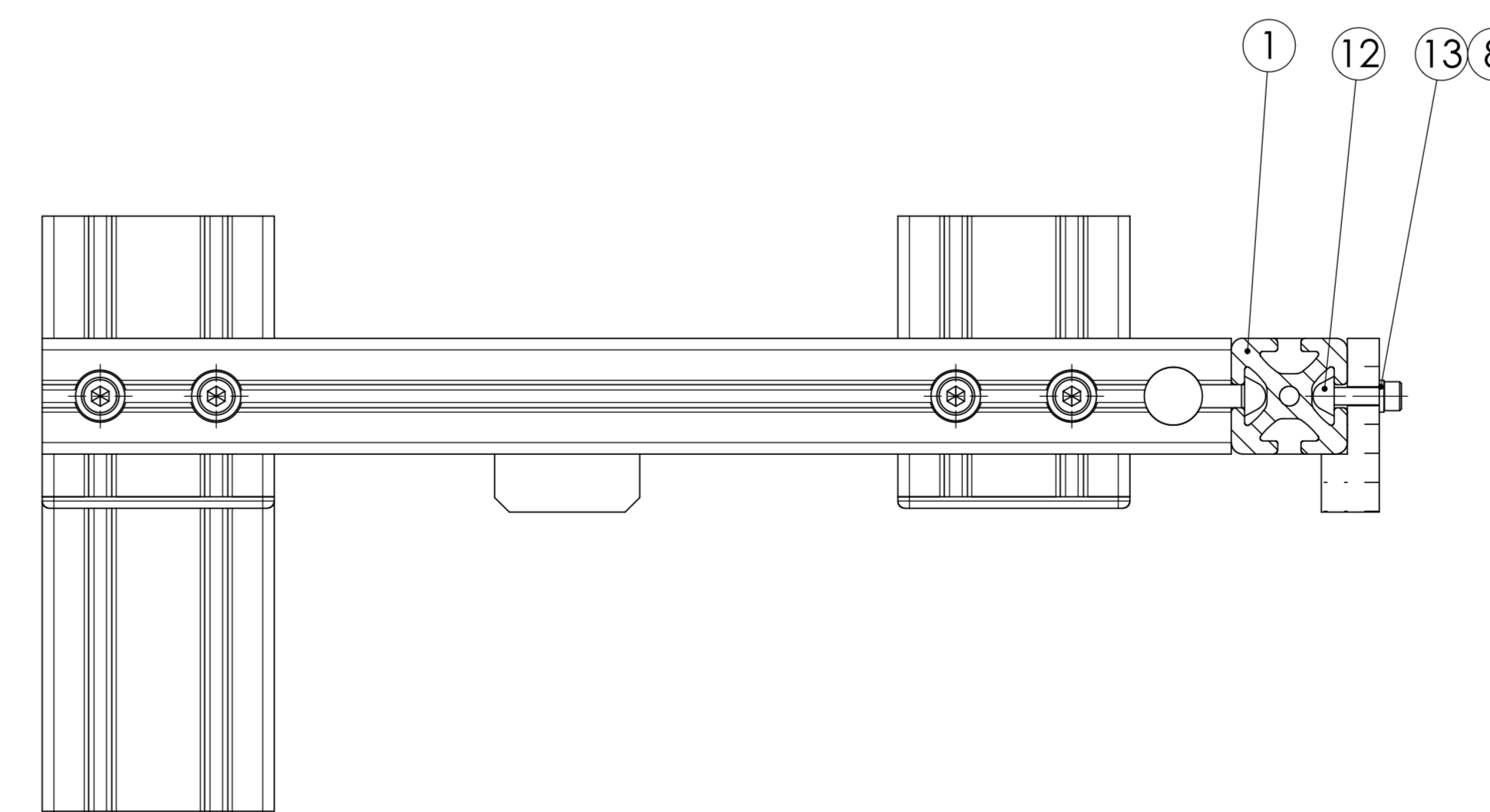
B-B (1 : 2)
