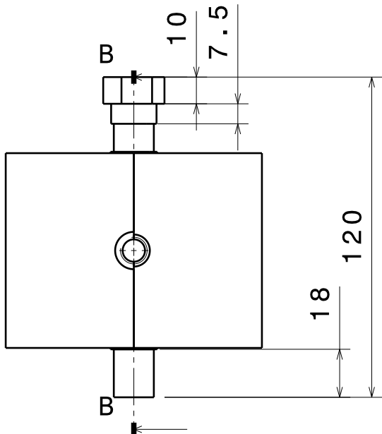
Seitenansicht rechts Maßstab: 1:2
