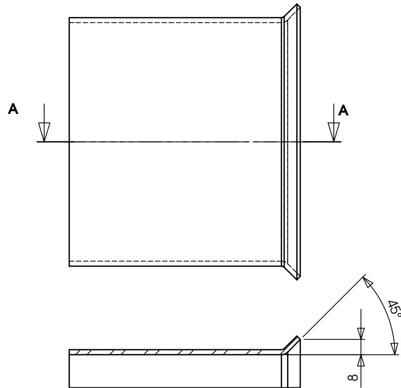
SCHNITT A-A
