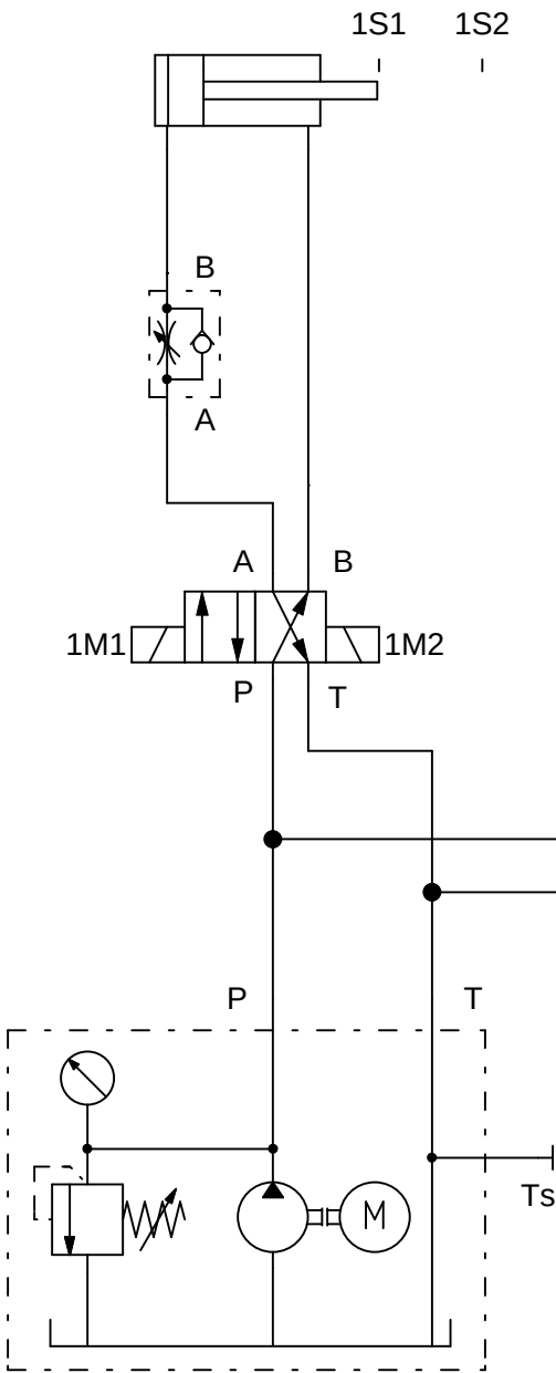
Spannzylinder 1A1
