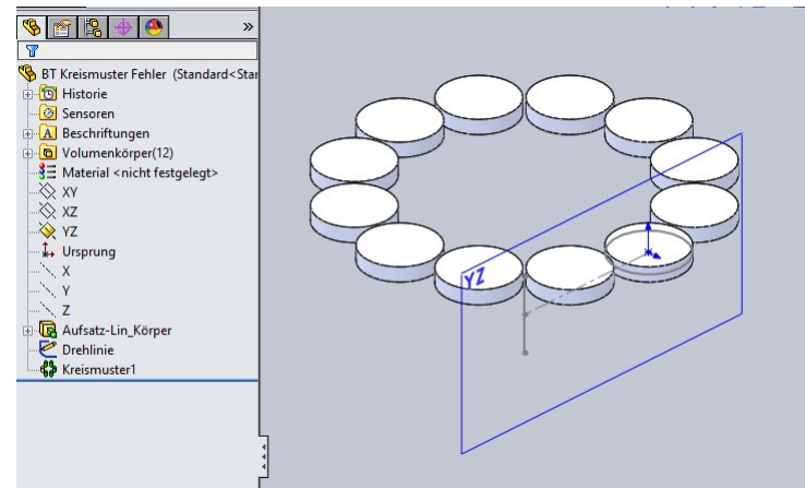
Drehachse wird an falscher Position verwendet.
