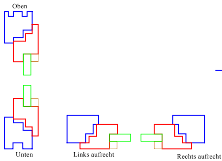
1 Schritt / erstellen der Schnitte im Detail
