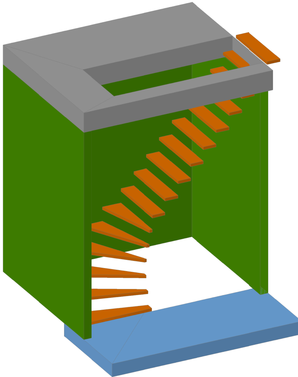
Treppe rechts laufend 1/4 gewendelt, Isometrie Maßstab 1 : 25 V3
