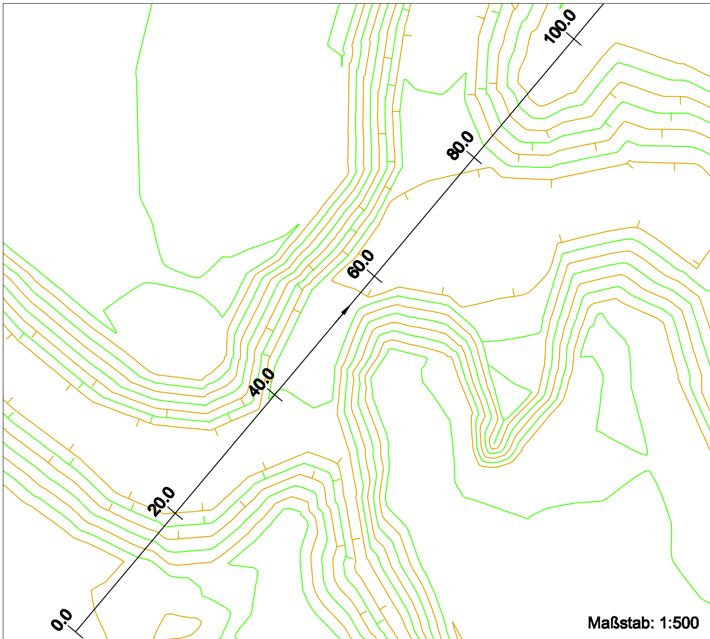
Höhenplan Systemschnitt Mitte Altwasser
