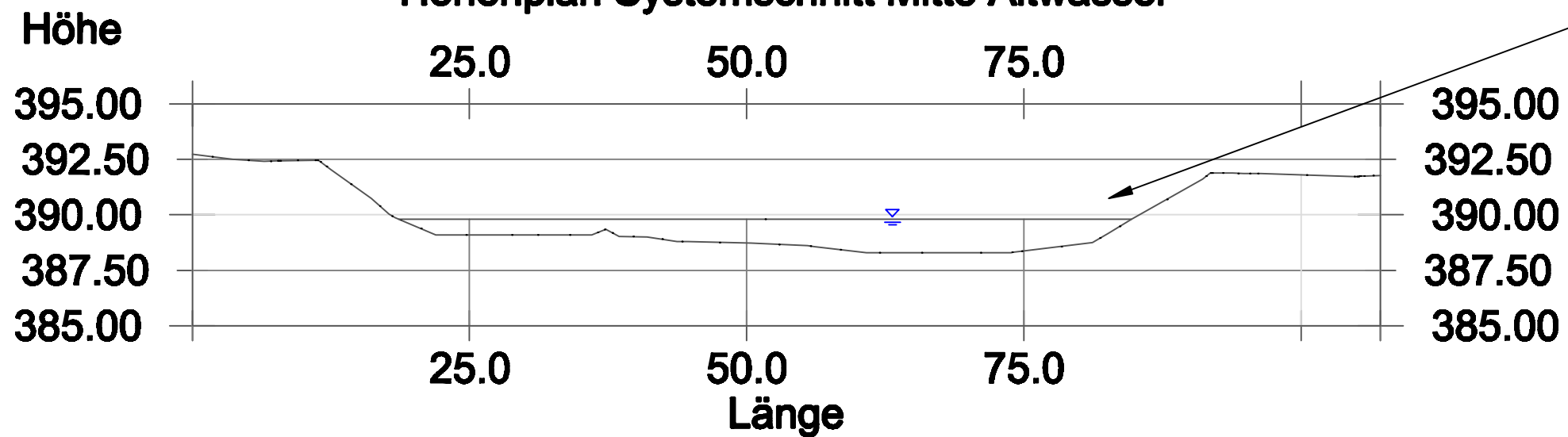
Höhenplan Systemschnitt Mitte Altwasser
