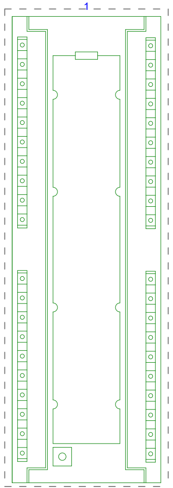
# SPS\Siemens\S7 300\SM 331 AI 8 x 13 Bit.ema Analogeingabe SM 331 8 AE 13 Bit Frontstecker 40-polig B x H: 40 x 125 mm Schaltschrankaufbau Variante A 2013-02-22 HKA
