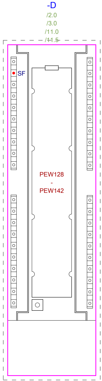
# SPS\Siemens\S7 300\SM 331 AI 8 x 13 Bit.ema Analogeingabe SM 331 8 AE 13 Bit Frontstecker 40-polig Allpolig Variante A 2013-02-22 HKA
