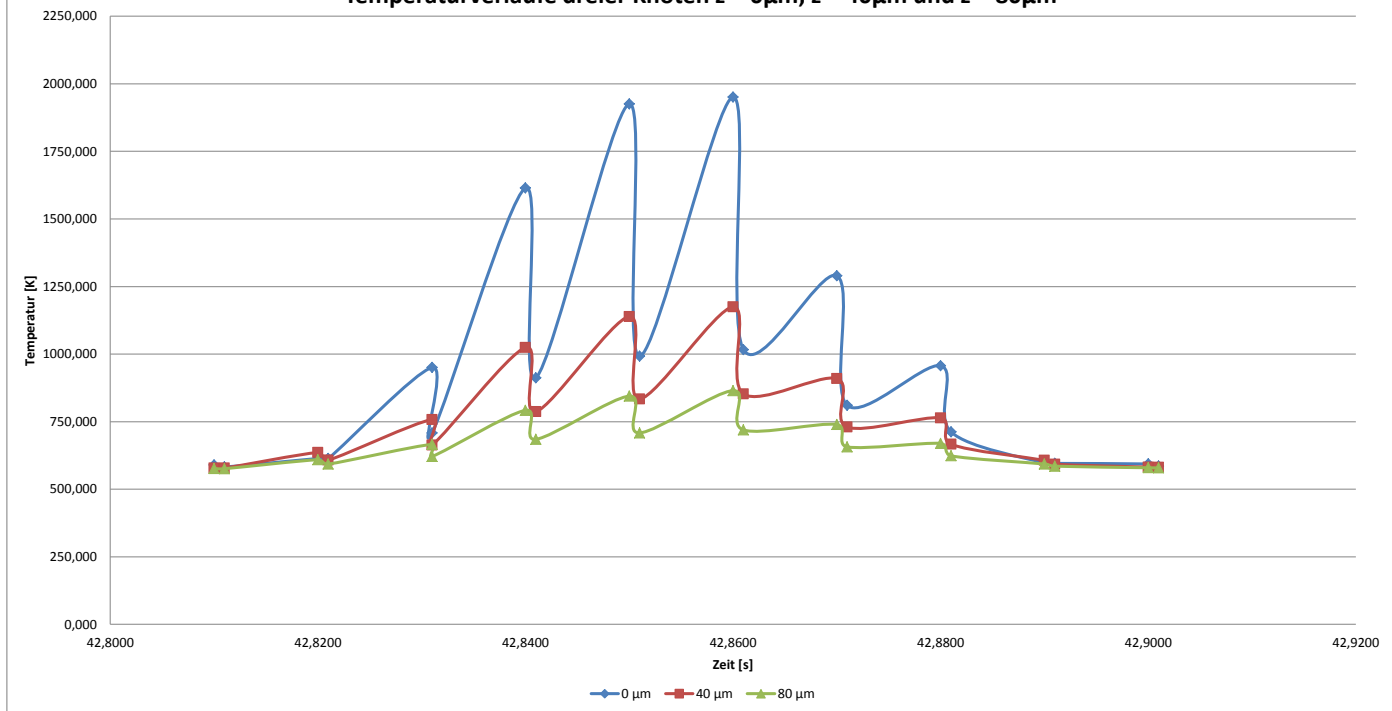
Temperaturverläufe dreier Knoten z = 0\mu\text{m} , z = 40\mu\text{m} und z = 80\mu\text{m}
