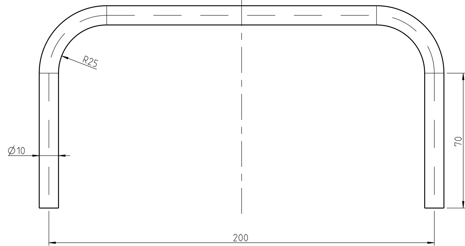
19 Ziehgriff
