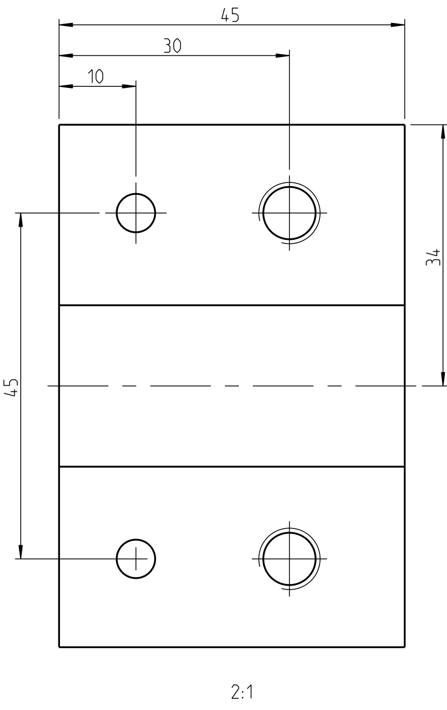
7 Halter unten
