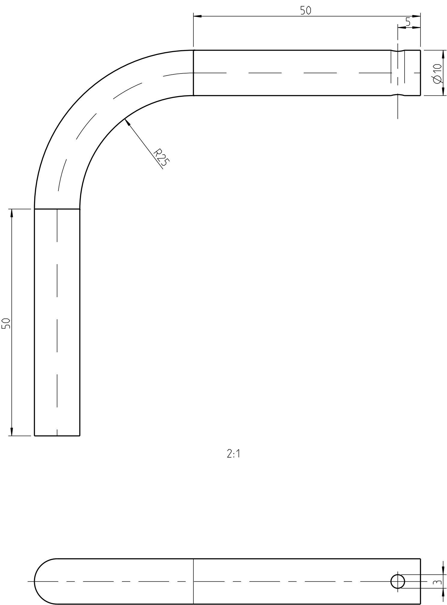
1 Absteckgriff
