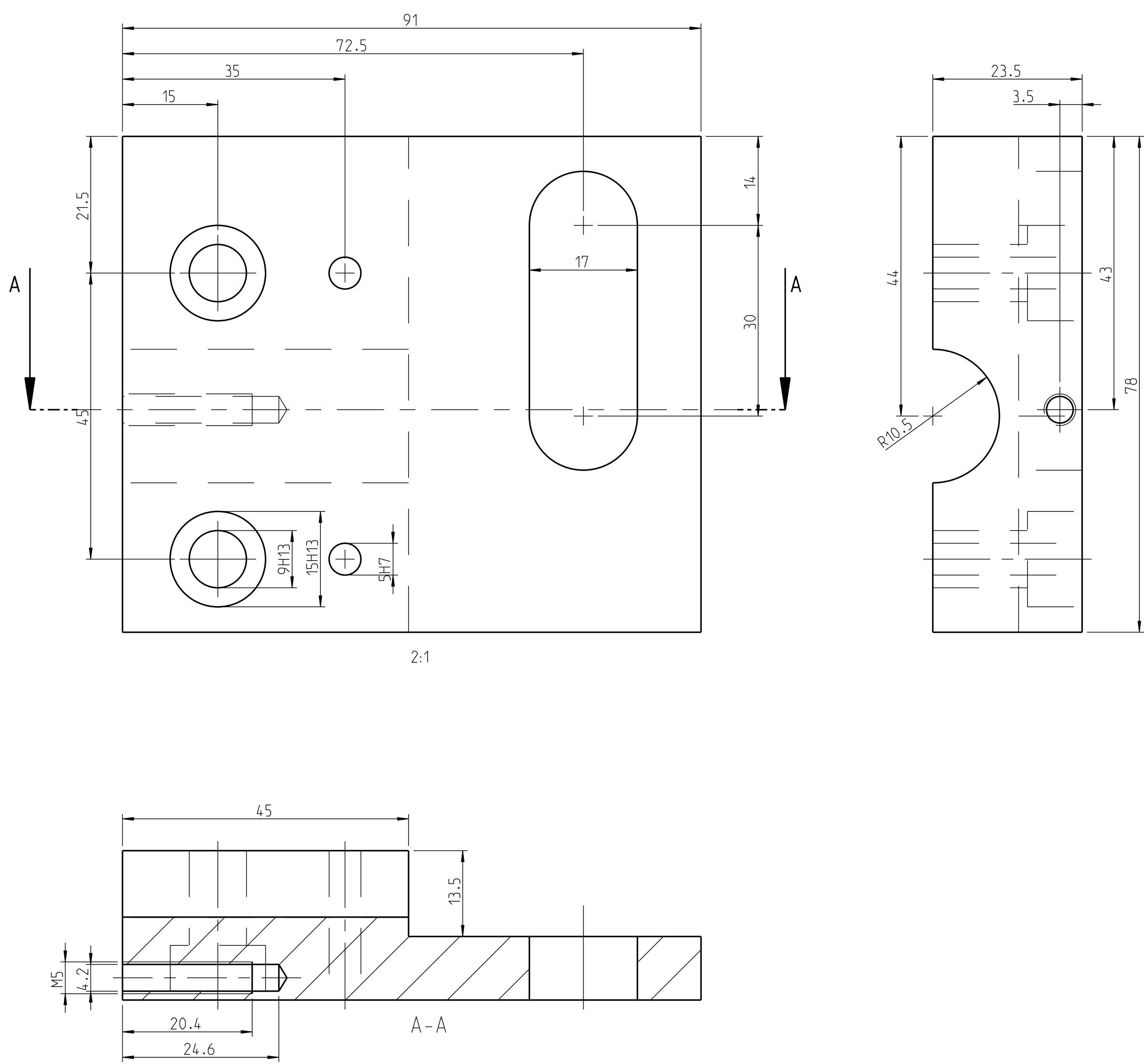
5 Halter oben
