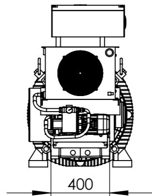
Motor M24
