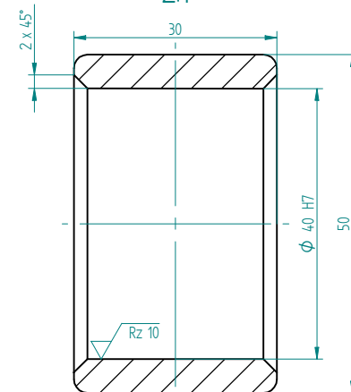
Schnitt B-B 2:1
