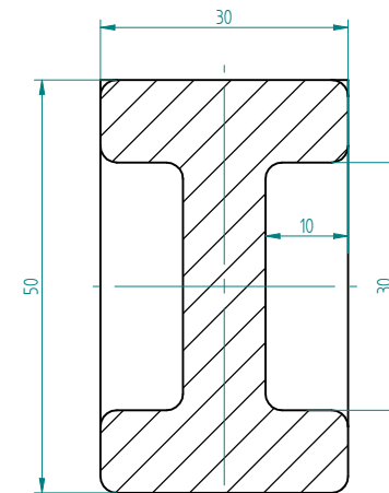
Schnitt A-A 2:1
