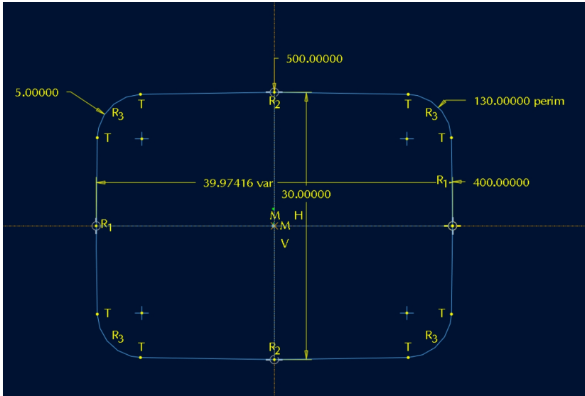
Skizze-Führungskurve-WF-2
