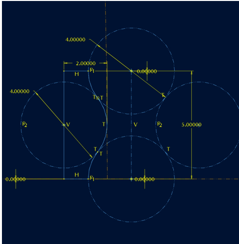
Skizze-Profil-WF2
