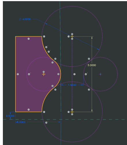
Skizze-Profil-Creo-7
