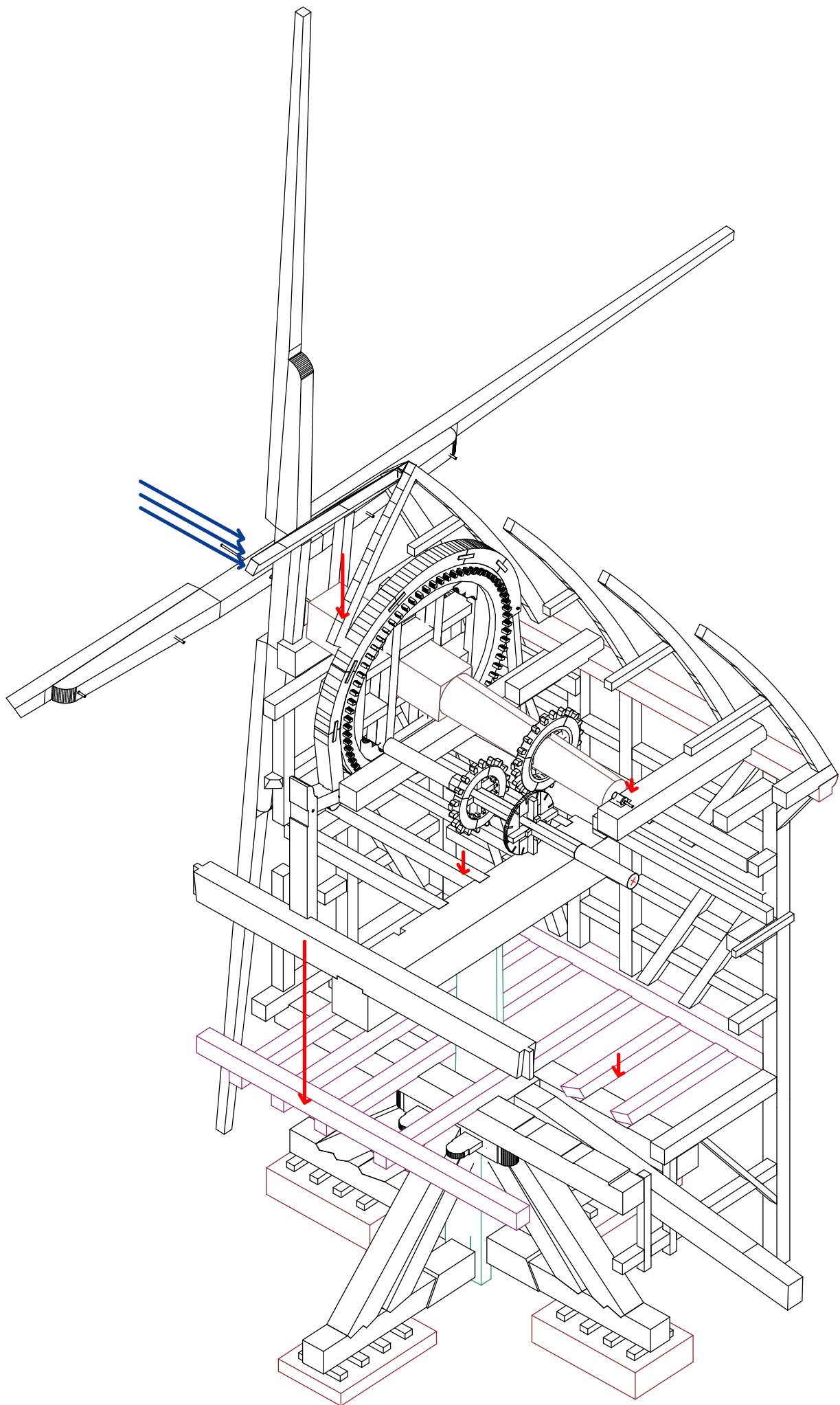
Mühle mit gehendem Werk und Lastverhältnissen
