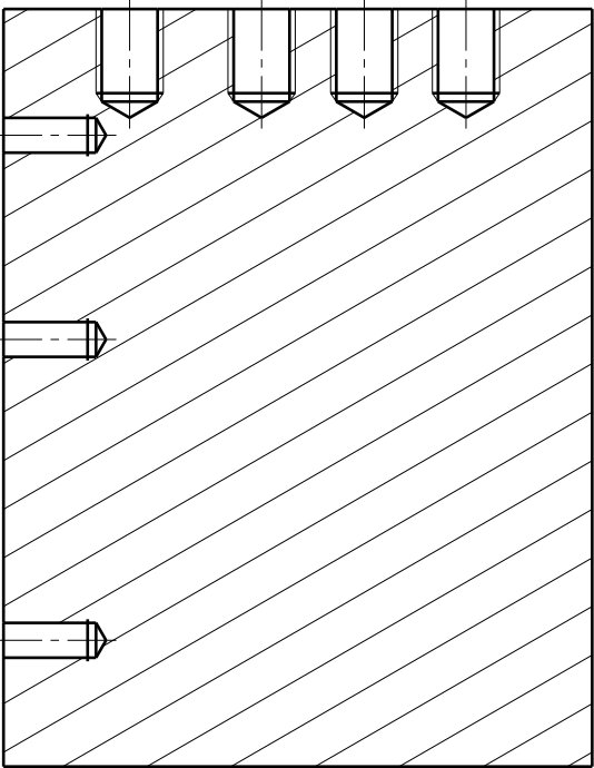
Schnittansicht F-F Maßstab: 1:1
