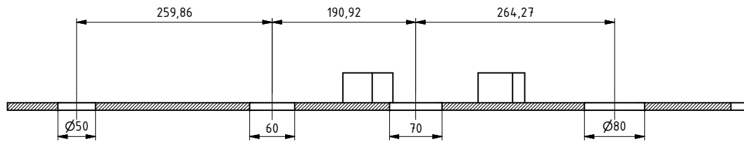
A-A Inventor 2010, Schnittmethode "Ausgerichtet"
