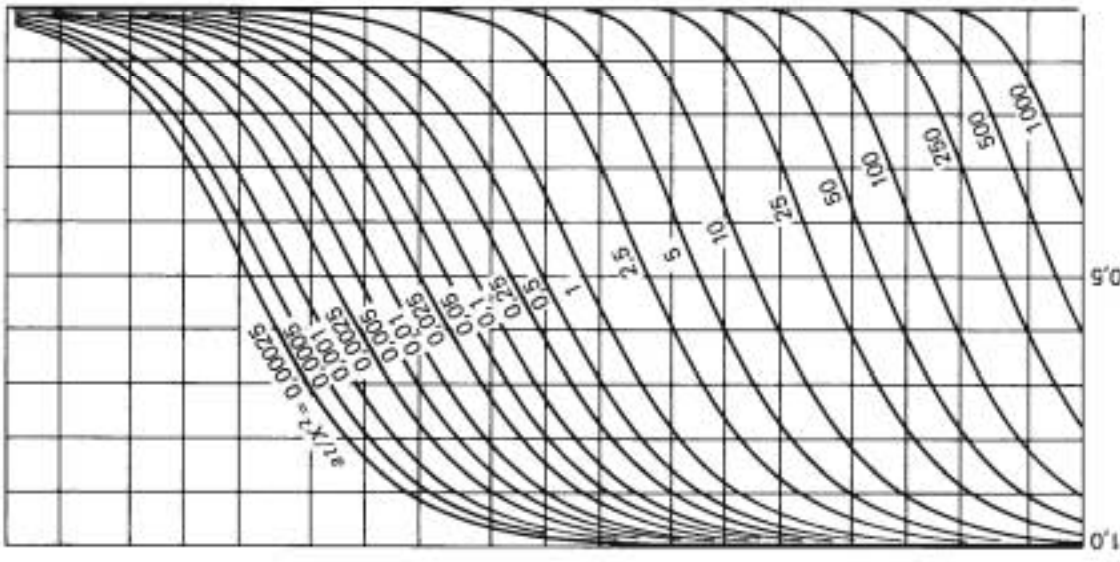
Normierte Temperatur \Theta_0 der Plattenoberfläche
