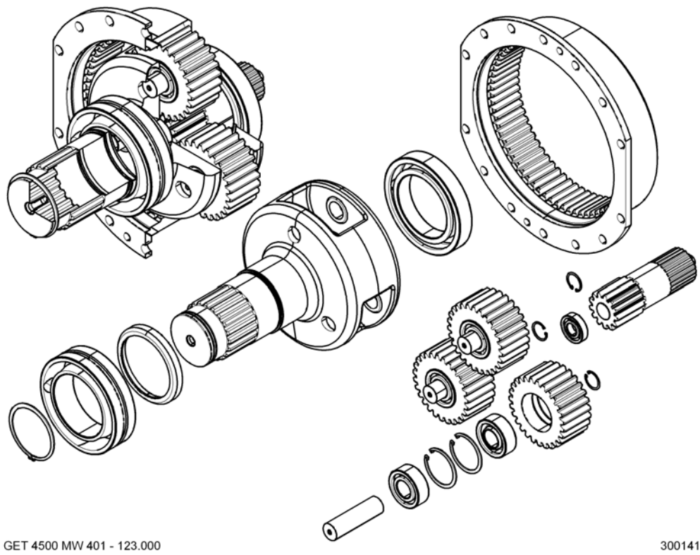
Fig. 0-4 Rohdaten aus 3D-CAD (Beispiel 1)
