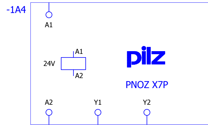
Gerätekasten Hauptfunktion
