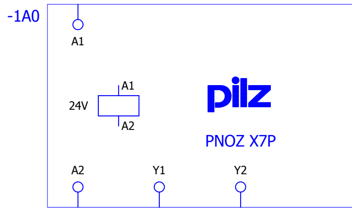
Spule Hauptfunktion
