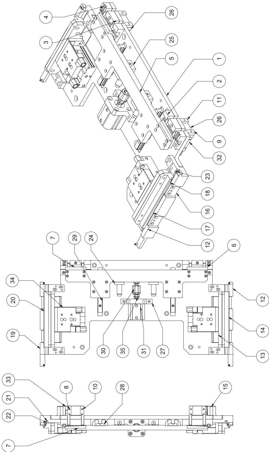
Abb. 5.3/11 Baugruppenzeichnung
