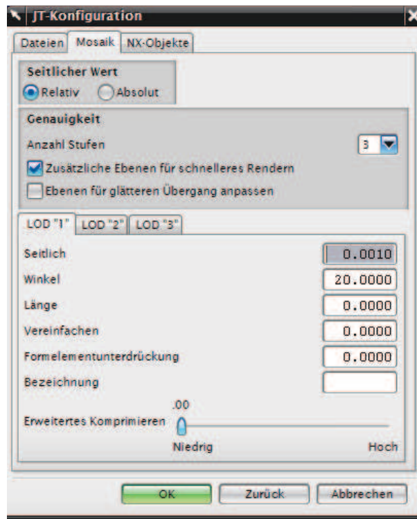
Seitlich (Chordal)
