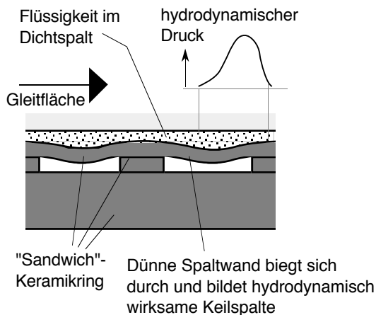
Bild 33 Elasto-hydrodynamische Druckerzeugung durch nachgiebige Dichtspaltwand
