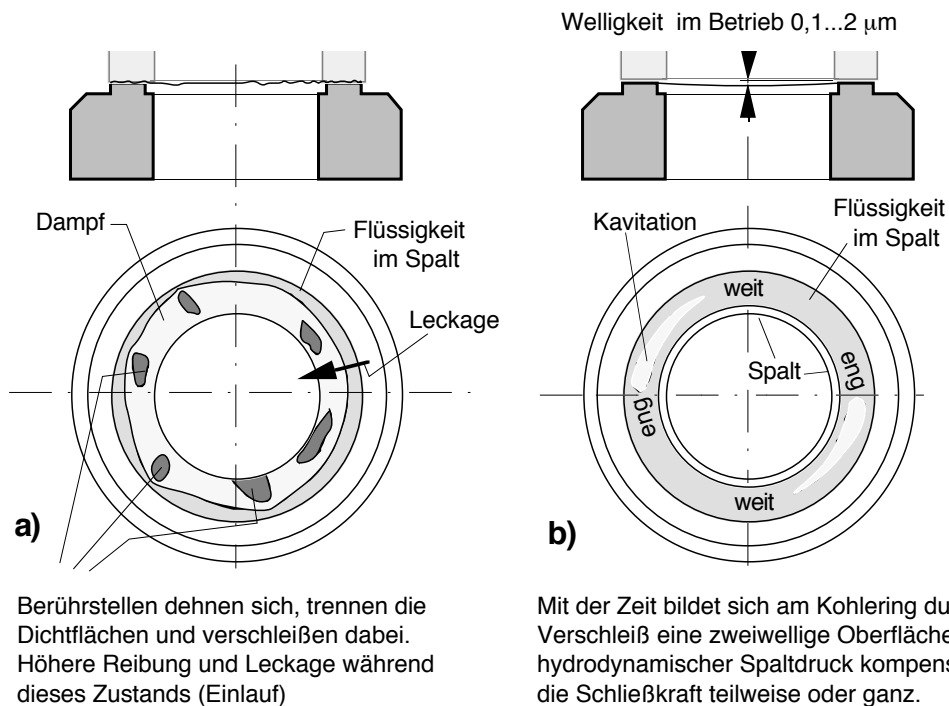
Bild 17 Veränderung der Gleitfläche eines Kohlegraphit-Gleitlings beim Einlauf
