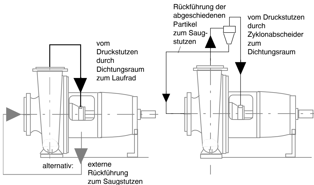
Bild 25 Zirkulation des Pumpenförderstroms durch die Dichtkammer von Kreiselpumpen zur Stabilisierung der Gleitringdichtung
