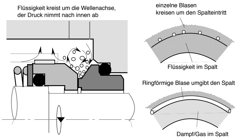
Bild 19 Dampf- oder Gasblasen in der Dichtkammer
