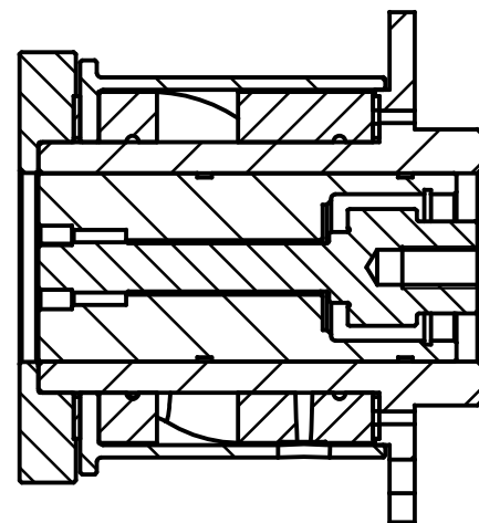
Schnitt A-A
