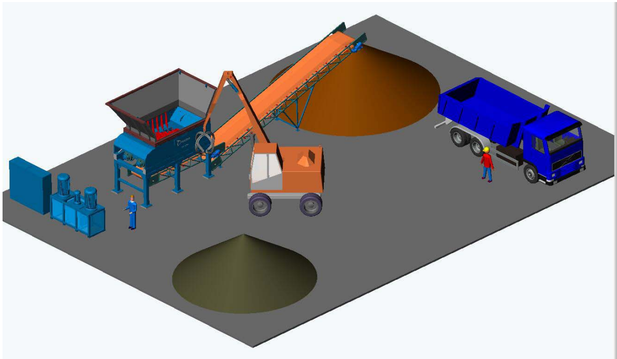
TPS 50 für Metso Lindemann GmbH, Düsseldorf
