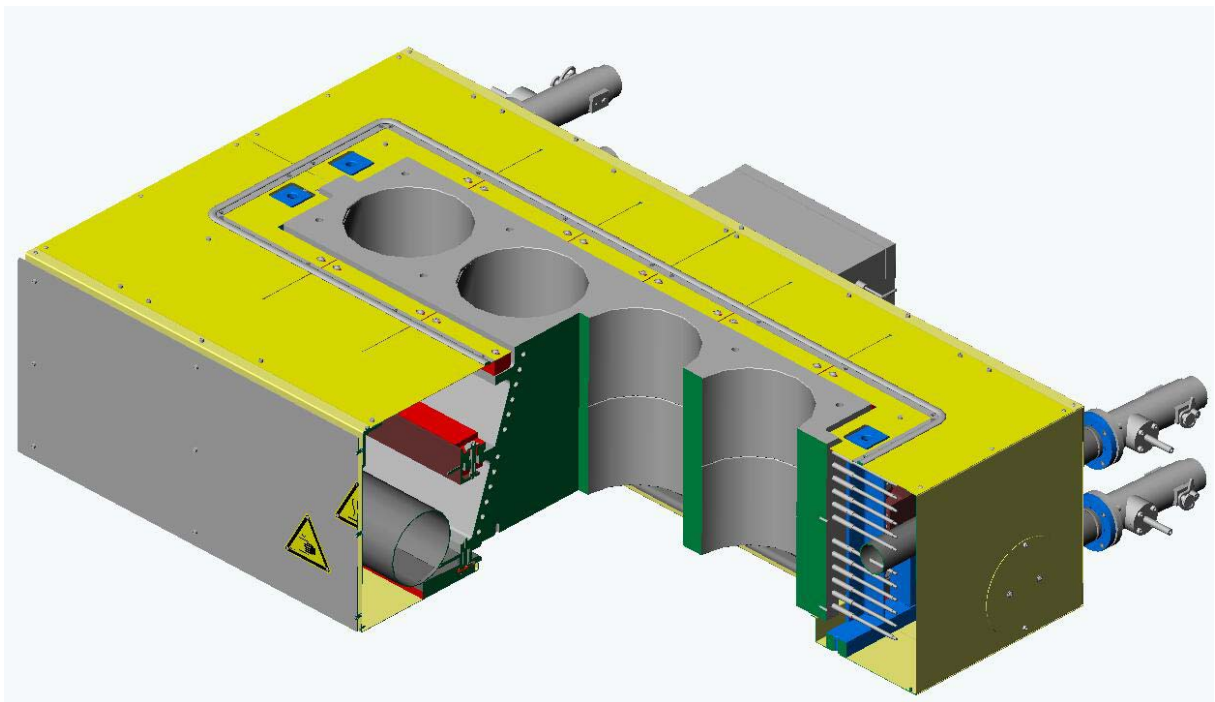
Nacherhitzer für Barmag AG, Remscheid
