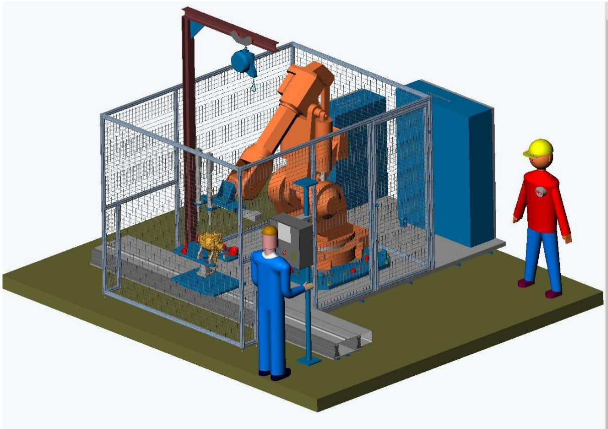
Roboterstation A230, Getriebedeckel verschrauben für ZF Gotha
