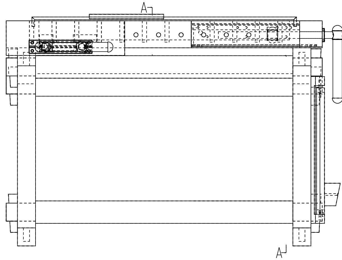
Vorderansicht
