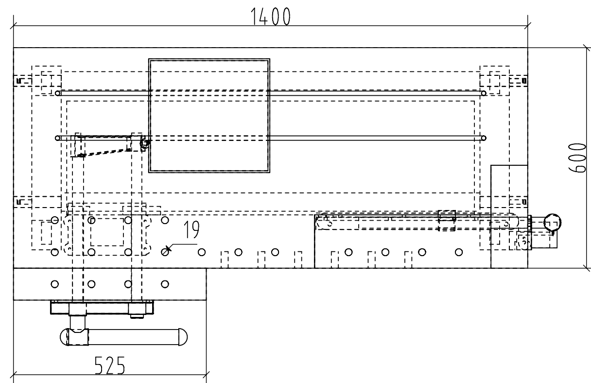
Draufsicht
