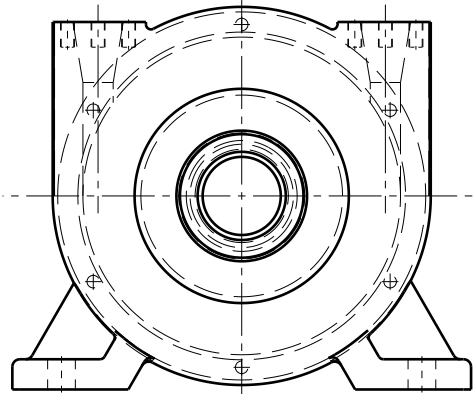
Vorderansicht Maßstab: 1:3
