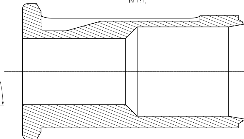
Schnitt A-A (M 1 : 1)
