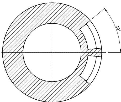
Schnitt C-C (M 1 : 1)
