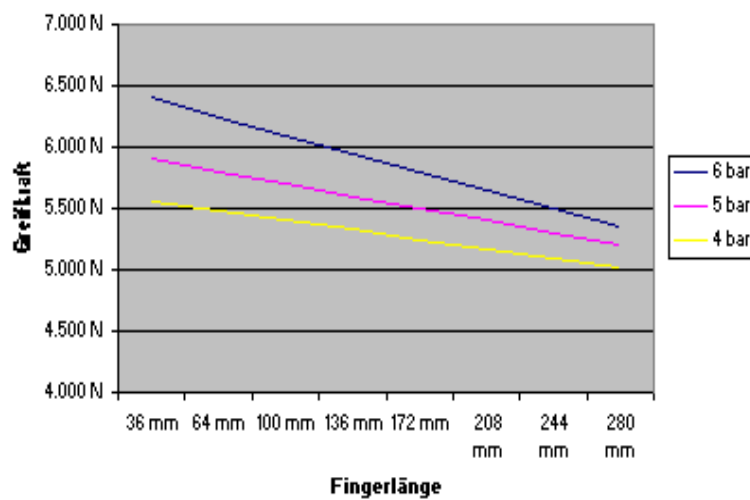
Fingerlängendiagramm WG-160
