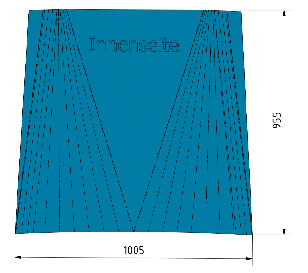
Uebergang-Abw-02 ( 1 : 10 )
