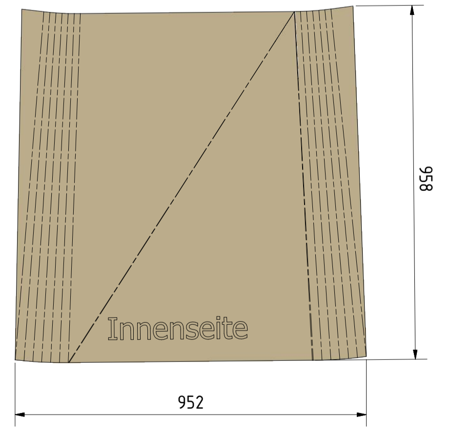
Uebergang-Abw-01 ( 1 : 10 )
